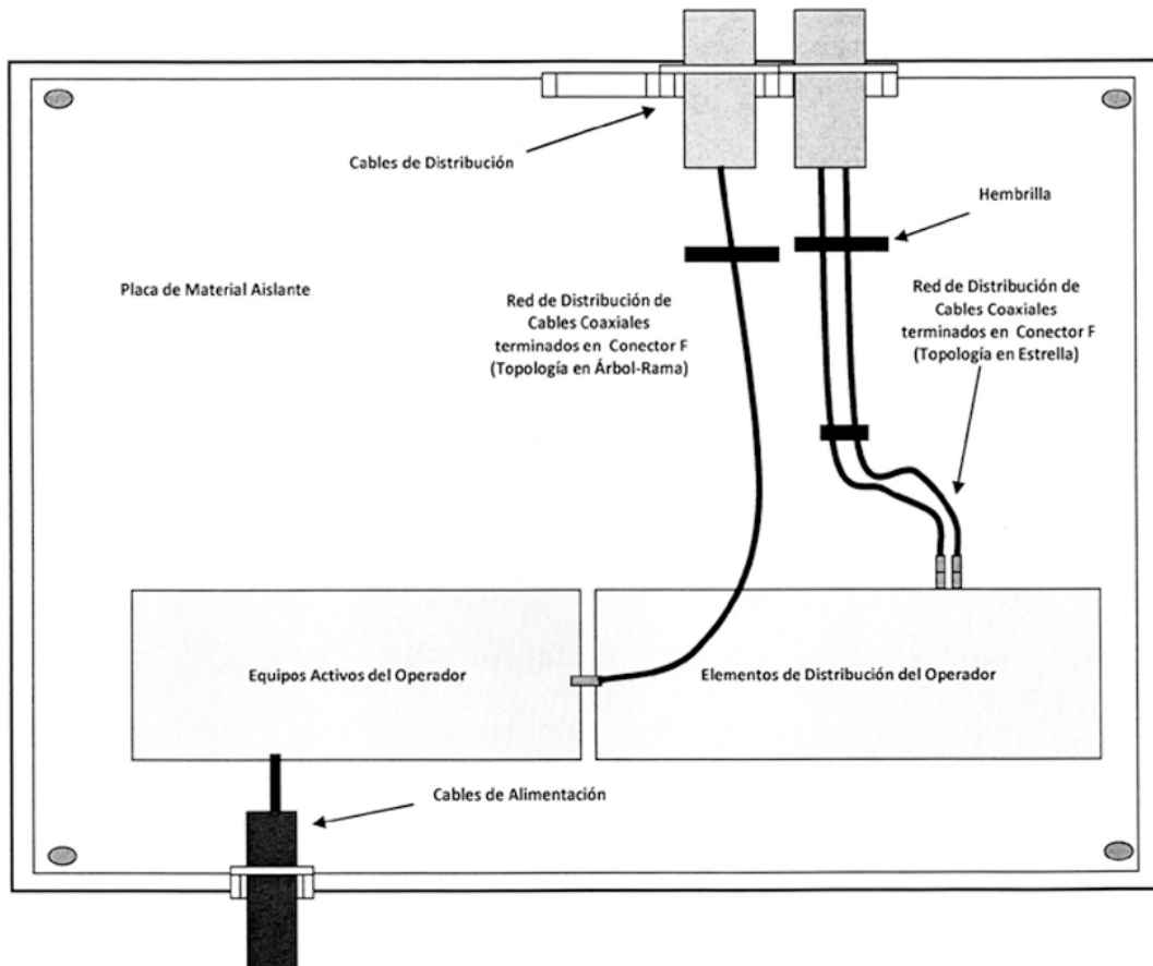
Apéndice 6: Punto de Interconexión de la Red de Cables Coaxiales
