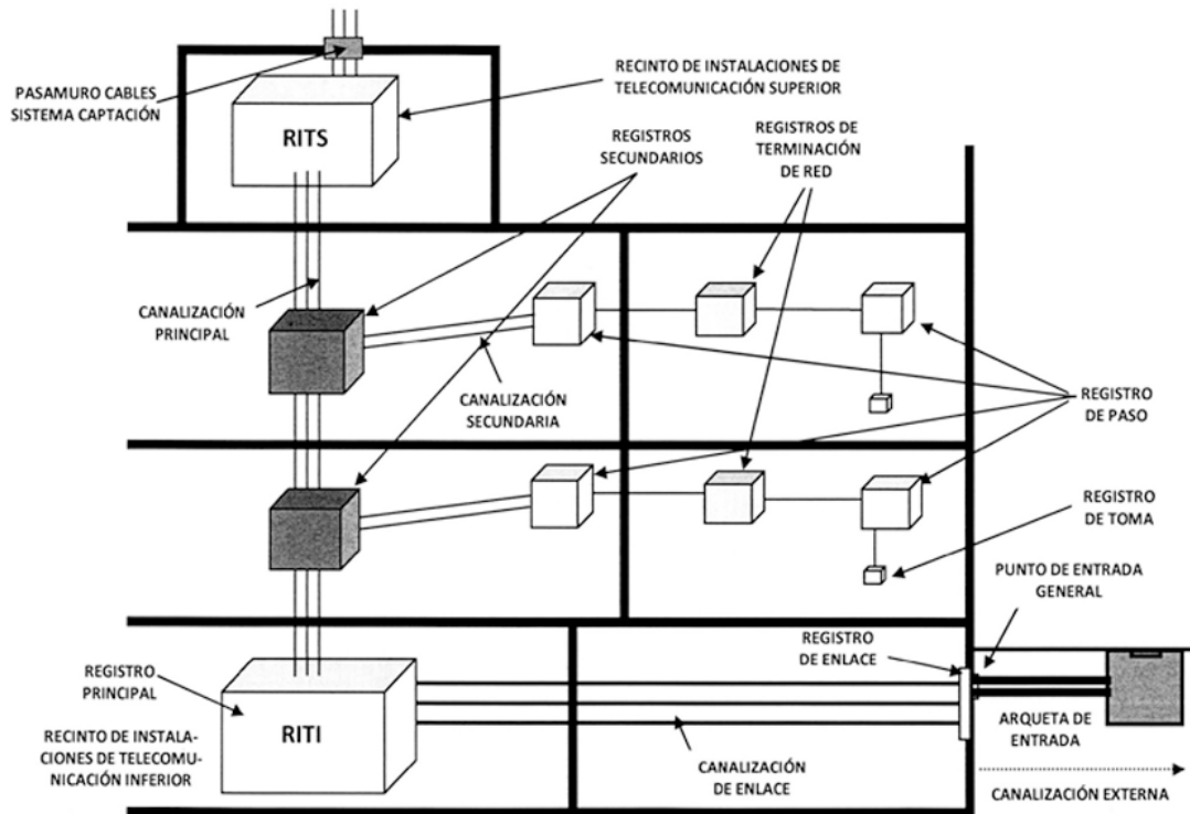
APENDICE 1: Esquema general de una ICT
